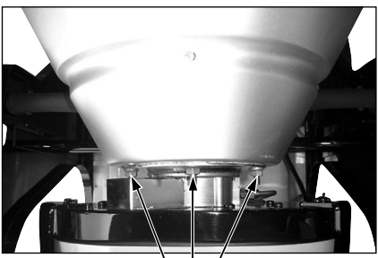
Desenrosque las tres tuercas y extraiga la unidad del quemador.
