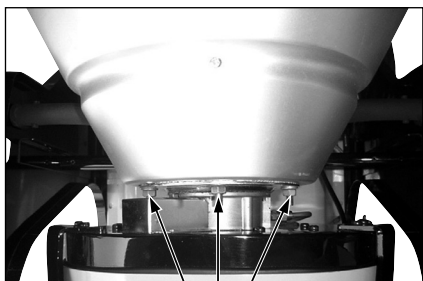
Die drei Muttern lösen und die Brennereinheit abnehmen
