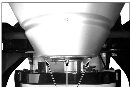
Dévissez trois écrous et déposez l'ensemble brûleur
